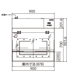
外形図
